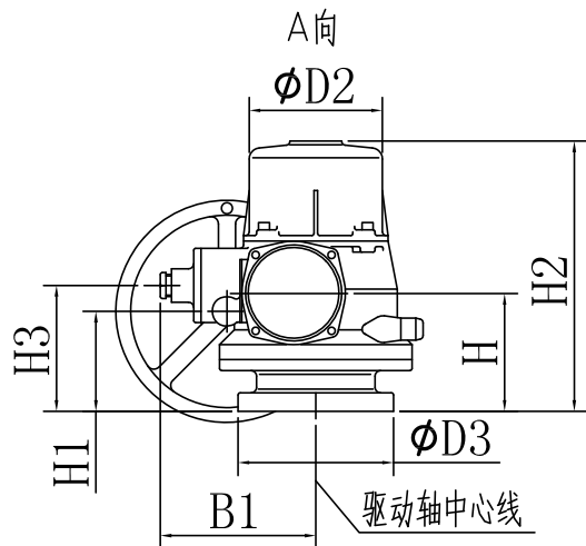
QBR3~QBR5系列外形尺寸
